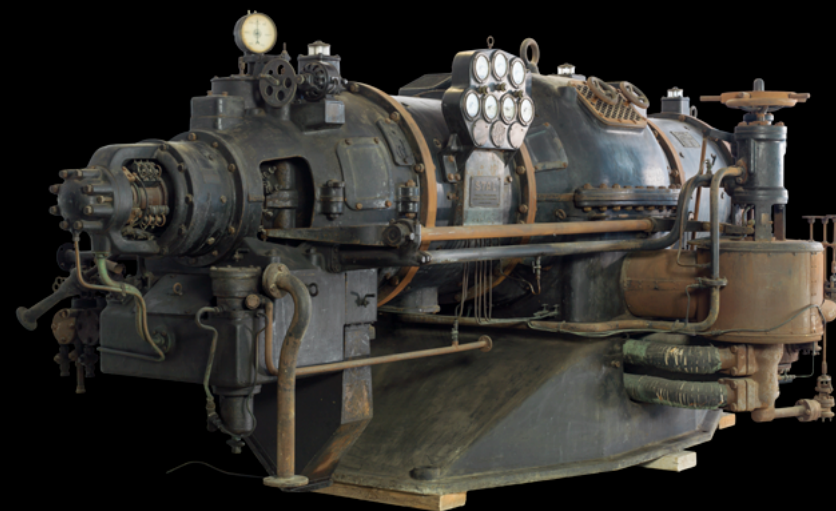
Turbogenerador de vapor, ASEA (1931)
